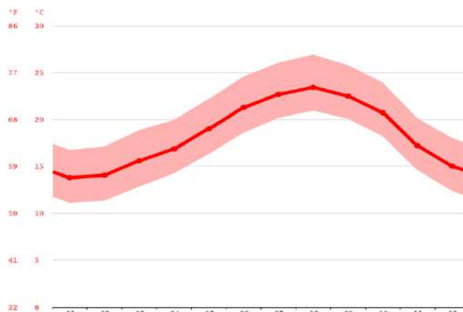
Figure 20: COURBE DE TEMPÉRATURE SIDI BOUZID
