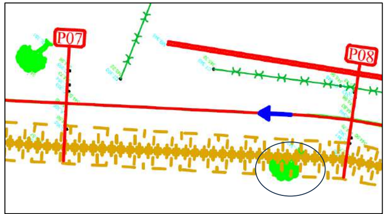
Figure 15: Extrait -Tracé en plan APD
