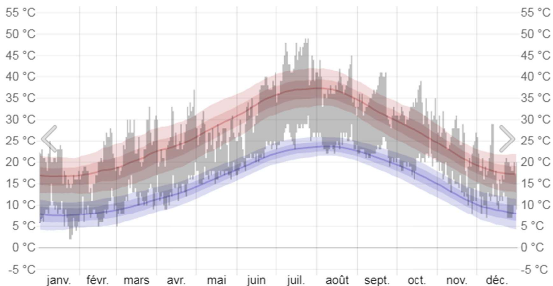
Graphique 1: Températures max et min moyennes mensuelles (°C)
