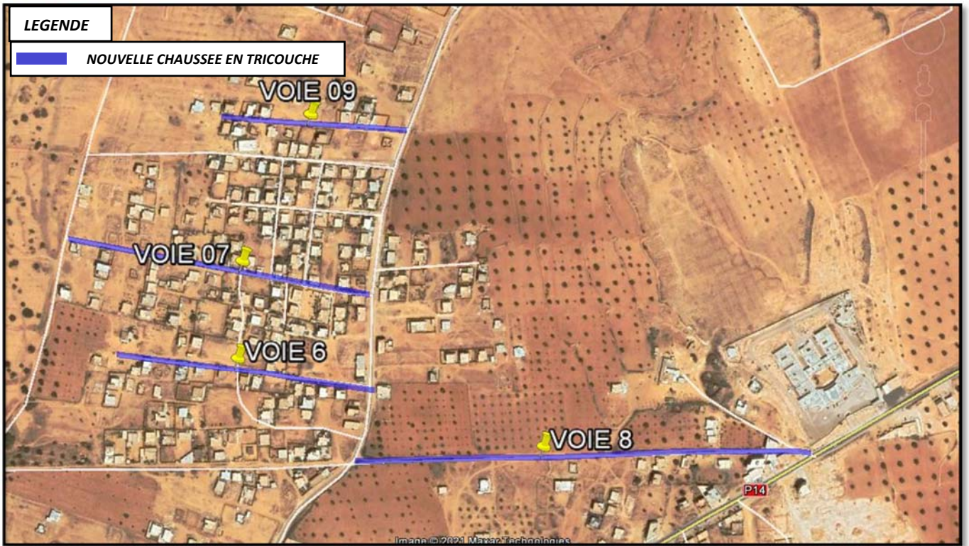
Plan d'intervention voiries : Cité ARARMA
